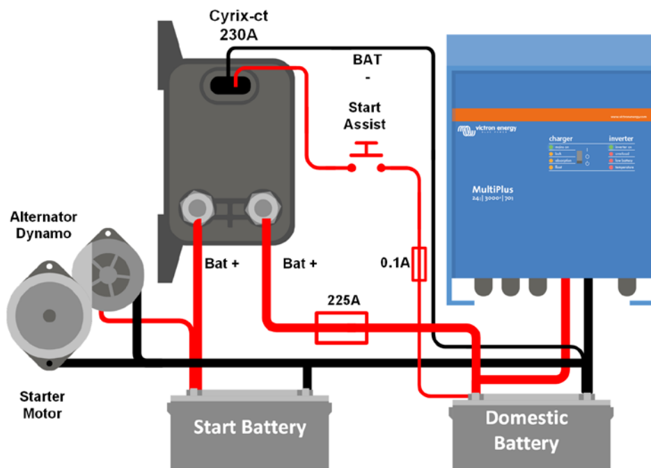
Cyrix-ct 12/24-230: esquema de conexión
